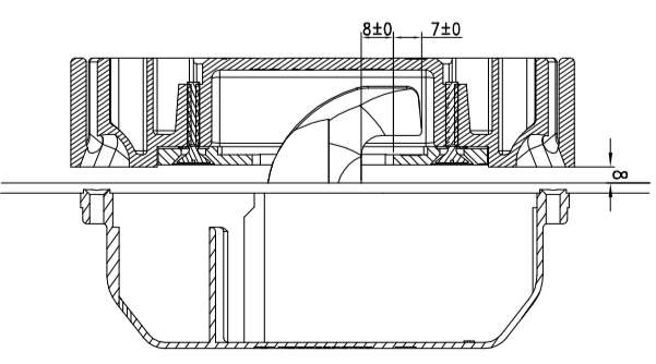
Detail Sluithaad in sluitkorn
