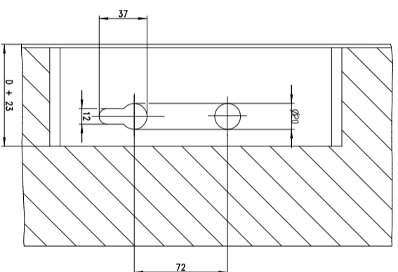
Frezing voor de Hoofdstotkast
