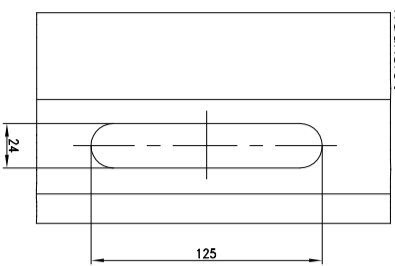
Frezing in het kozijn voor sluitkom hoofdstot
