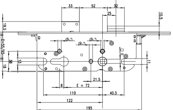
Maatvoering hoofdstotkast
