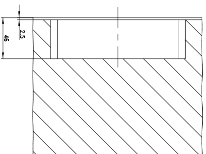
Frezing voor bijzet slotkast voor sluithaak
