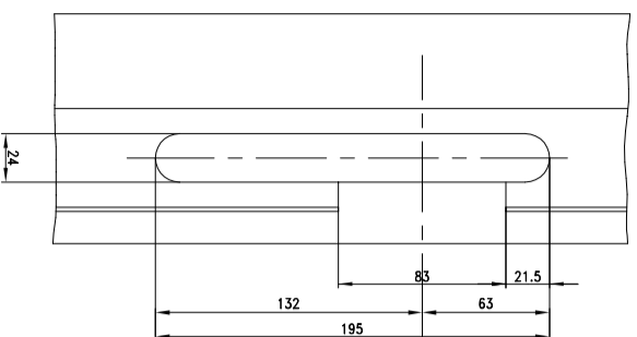
Frezing in kozijn voor sluitkom hoofdstot
