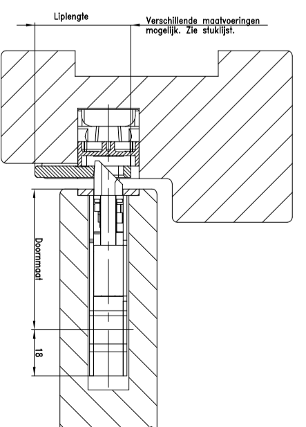
Doorsnede deur en kozijn
